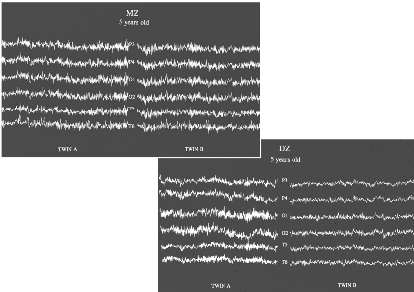
Figuur 6. Electro-encefalogrammen (EEG) van eeneiig MZ- (bovenste) en twee-eiig DZ- (onderste registratie) tweelingen.
